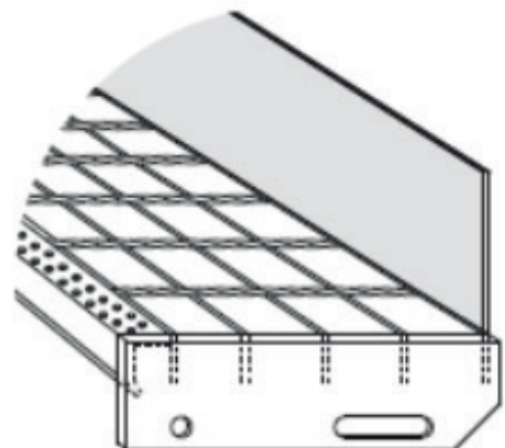
Illustrasjon av sparkeplate for trinn.
