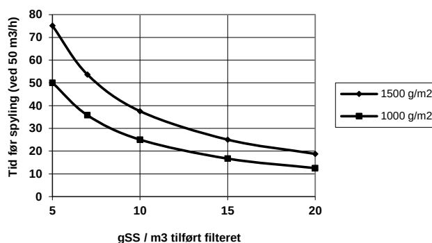
Figur 4. Driftstid før spyling som funksjon av tilført mengde SS (ulike lagringskapasiteter).
