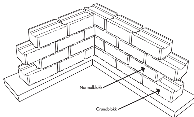
Bilde 9. Innvendig 90° hjørne.
