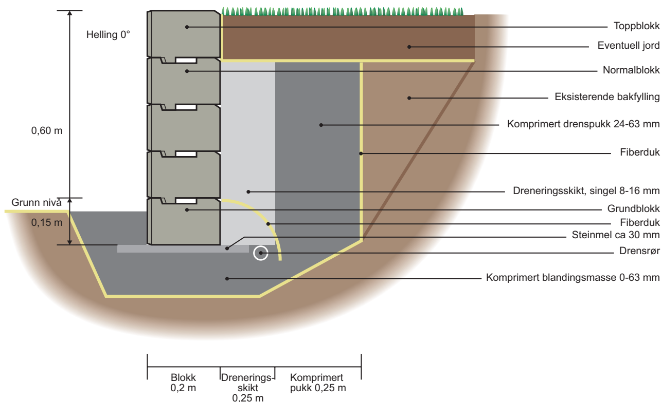
Bilde 1. Seksjonsteining for mur opp til 0,6 m.
