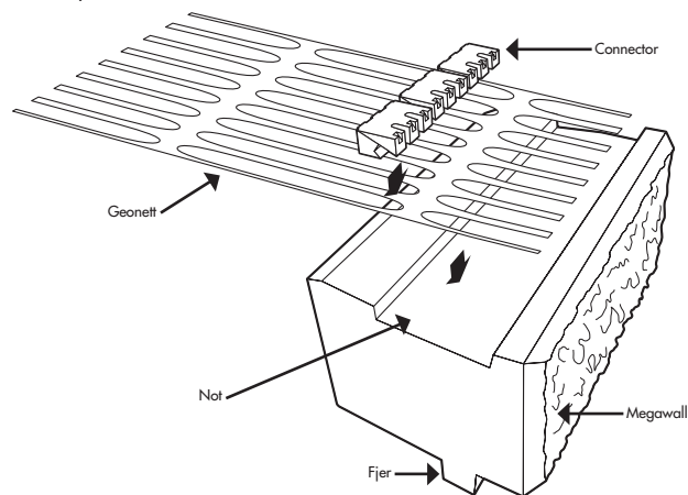
Bilde 4. Montering av Connector og Geonett.
