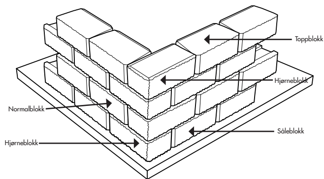
Bilde 9. Innvendig 90° hjørne.
