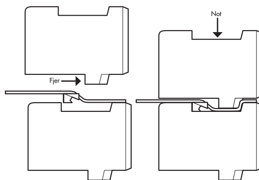
Bilde 4. Montering av Connector og Geonett.
