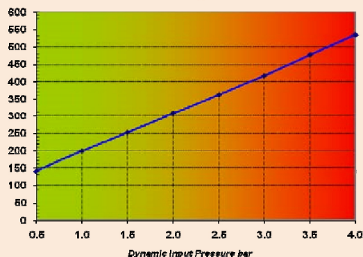
590HV Air Cap Air Flow
